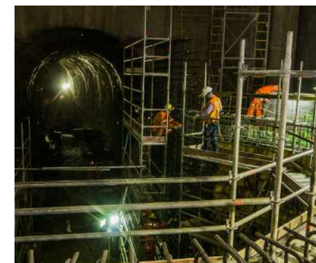
Alto Maipo está compuesto por dos centrales de pasada que generarán 531 MW y el agua que se utilice en la generación de energía será devuelta en un 100% al cauce del río Maipo.
